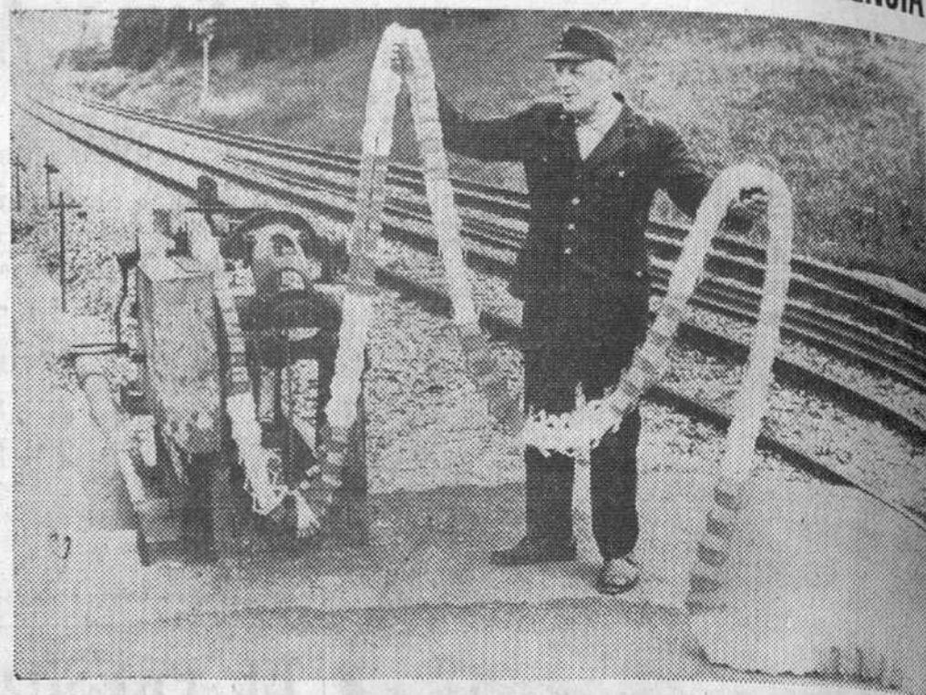
Para el caso de que las barreras de los pasos a nivel se estropeen, los ferrocarriles alemanes han concebido estas guarnaldas de plástico pintadas de blanco y de rojo, que en su interior llevan una cuerda de perlon para estabilizarlas. — (Foto Fiel)
