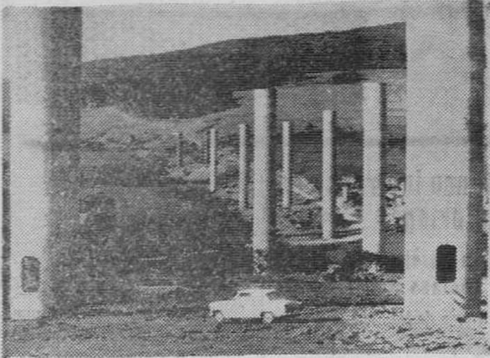
En la autopista Hamburgo-Bad Hersfeld-Munich, se está construyendo un puente que tendrá, una vez acabado, una longitud de 800 metros, para lo cual se están levantando 13 pilares de hormigón armado, con una altura de 50 metros. Este es el estado actual de las obras, que aparecen ante el visitante como extraños árboles crecidos junto al bosque. — (Foto Fiel)
