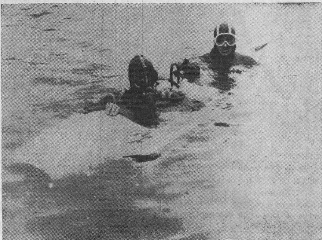
En aguas del Danubio, cerca de Viena ha sido presentado un submarino de bolsillo, el "Sea Shark II", que es idéntico al utilizado por el agente secreto James Bond en los films de sus aventuras. Tiene capacidad para dos personas y puede realizar inmersiones hasta 40 metros, consiguiendo una velocidad de 9 kilómetros por hora. Construido en fibra de vidrio, tiene una longitud de 3,70 metros. En la foto vemos un momento de su presentación. — (Foto Fiel)
