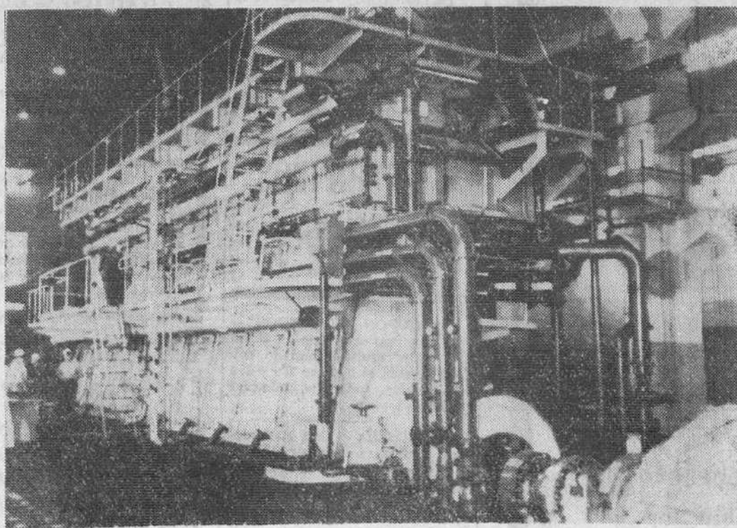
Valencia. — El «Manises Sulzer», el mayor motor por potencia de cilindros construido en España, ha sido sometido hoy a las pruebas oficiales en la factoría de Manises. — (Telefoto Cifra)
