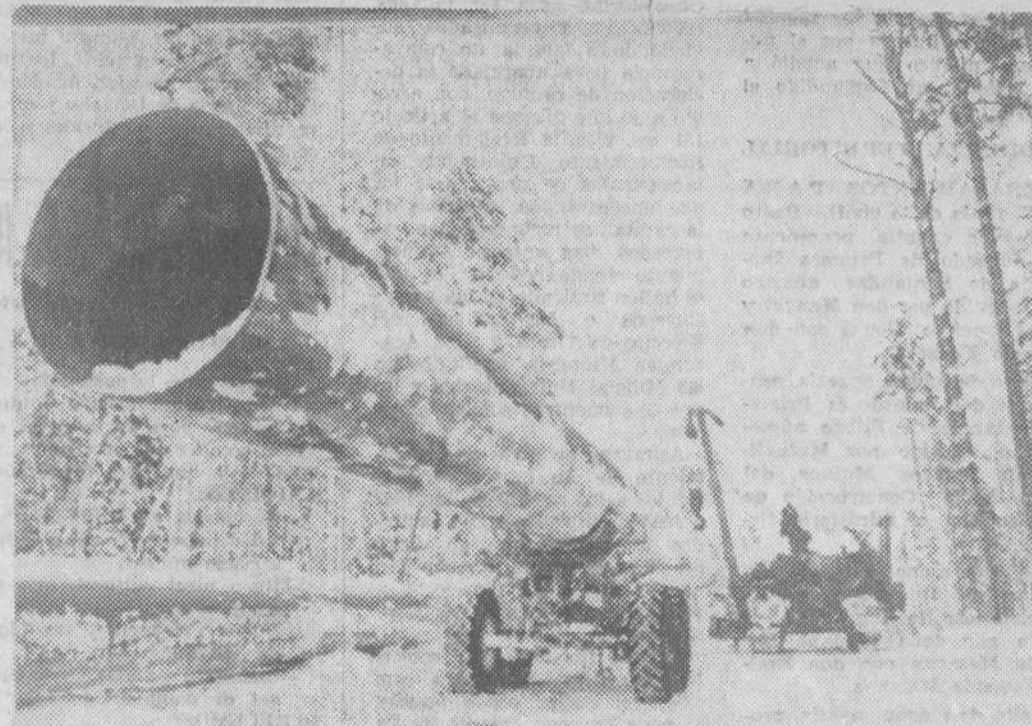
Entre la región de Berezo y la zona industrial de los Urales, se ha construido un gigantesco gasoducto de 500 kilómetros a través de La Taiga. Los tubos eran de 35 metros de largo y uno de diámetro. — (Foto FIEL)
