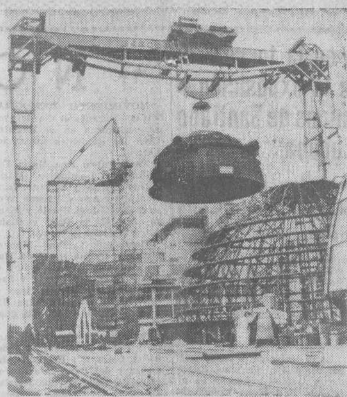
Una grúa "goliat" transporta para su colocación la parte esférica superior (400 toneladas), del reactor número 1 de la estación nuclear Wylfam, en Angelsey (Inglaterra). Será, una vez terminada, la mayor estación nuclear del Mundo y sus reactores están siendo construidos por la compañía inglesa Babcock & Wilcox. Producirá 1.180 megavatios y abastecerá al Noroeste del país en 1969. — (Foto Fiel)
