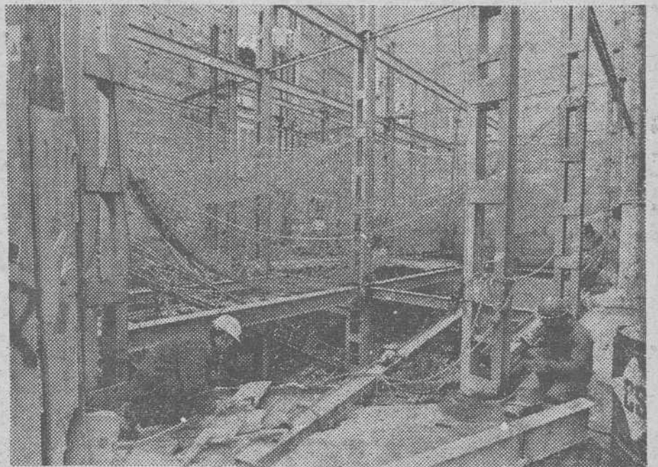
Para la prevención de los accidentes de trabajo, el problema esencial sigue siendo el de encontrar remedio a cada causa de accidente, como esta red que evita el golpe contra el suelo de los operarios dedicados al montaje de las vigas de la estructura de hierro. — (Foto EFE-FIEL).
