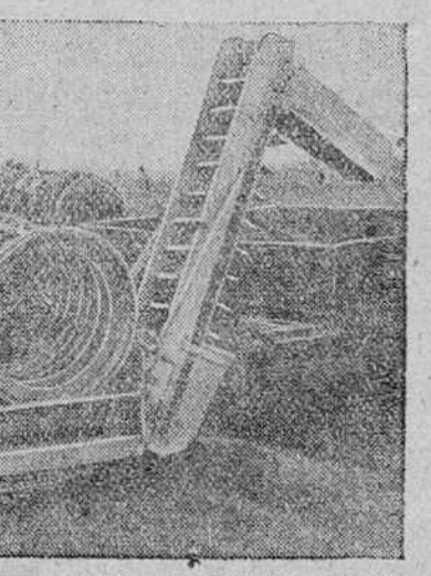
LONDRES.— NUEVA EXCAVADORA Y COSECHADORA DE PATATAS. ESTA MAQUINA AGRICOLA HA RESUELTO EL PROBLEMA DE RECOGER LAS PATATAS. VA MONTADA SOBRE UN TRACTOR DE 20 CABALLOS, Y CONSISTE PRINCIPALMENTE DE UN ROMPEDOR DE TERNONES DE TIERRA, UN CILINDRO LIMPIADOR Y UN ELEVADOR. LA FOTO MUESTRA UNA VISTA POSTERIOR DE LA MAQUINA EN LA QUE SE ADVIERTEN PERFECTAMENTE LAS PIEZAS PRINCIPALES MENCIONADAS. — (GALPE)
