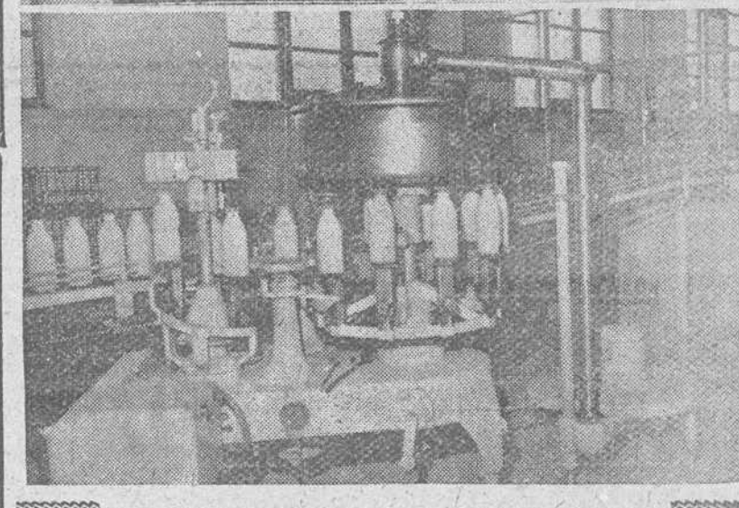
Tres aspectos de las instalaciones de la Central Lechera de Burgos, S. A., inauguradas y bendecidas ayer tarde; de arriba a abajo, los tanques isotérmicos para la leche, la esterilizador automática de botellas y una vista general de la sección de embotellado. — (Fotos "Fede")
