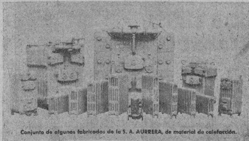
Conjunta de algunas fabricados de la S. A. AURRERA, de material de calefacción.
