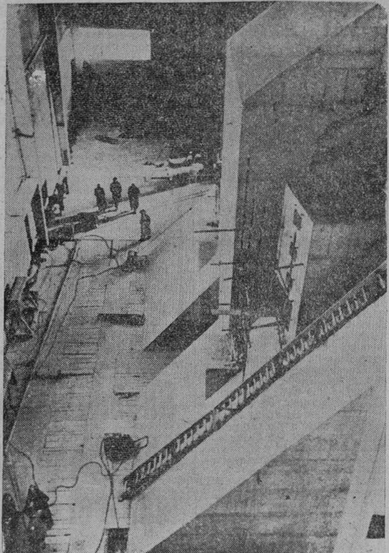
He aquí la parte oeste de la pila G-1 de Marcoule, que producirá 15 kilogramos de plutonio por año. Puede apreciarse la grandiosa protección de hormigón. — (Foto Gil del del Espinar)
