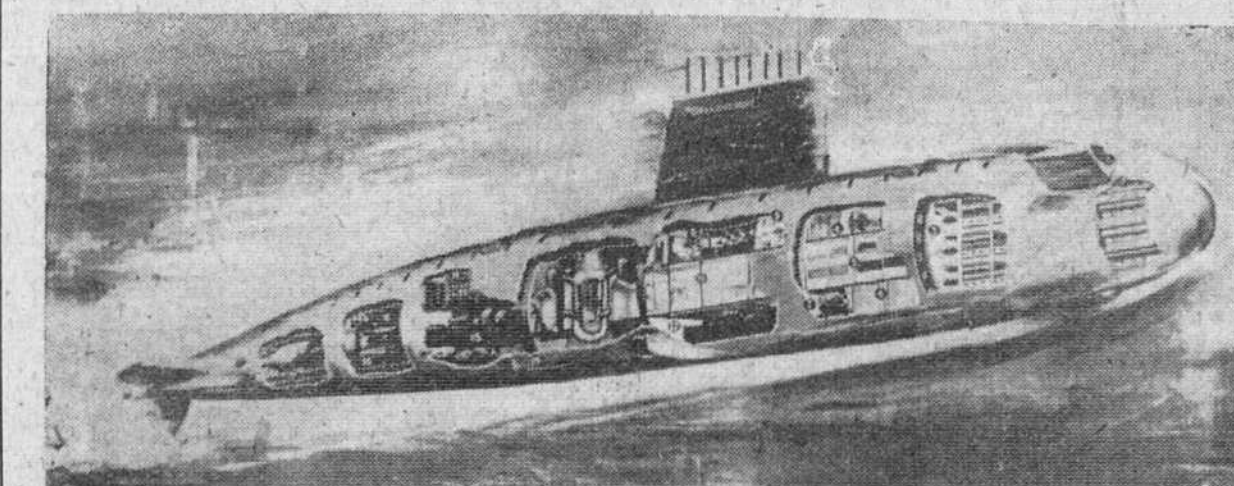
Londres.— He aquí un dibujo para mostrar la posición de los principales compartimentos del submarino nuclear británico "Dreadnought" que será botado el próximo día 12 en los astilleros de Barrow-in-Furness, con asistencia del duque de Edimburgo. La maquinaria que será instalada en su interior será similar a la del submarino atómico norteamericano "Skipjack".— (Foto Cifra)
