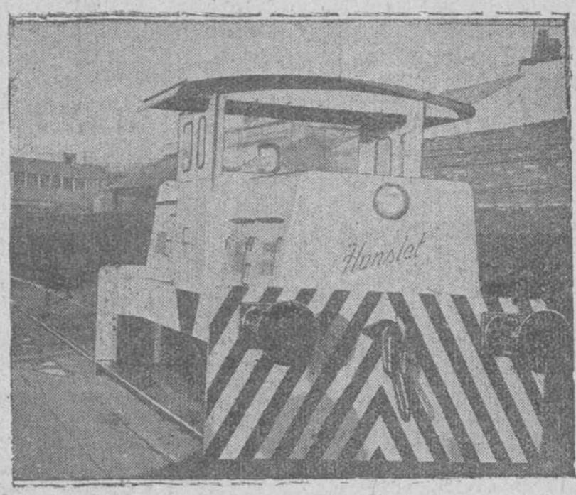
Esta locomotora Diesel, que se halla actualmente en servicio en Salisbury, (Rhodesia Meridional) es la última aportación británica para resolver los problemas de las maniobras ferroviarias. Está propulsada por un motor diesel que desarrolla una potencia de 71 h. p. Aparte de las posiciones usuales desde las cuales conduce el maquinista la máquina señala, una a cada lado de la cabina, la locomotora puede ser manejada mediante controles de botón desde las escaleras de ambos lados, lo cual evita la necesidad de que el maquinista vuelva a la cabina cada vez que tenga que efectuar una maniobra. Después de cambiar de agujas o de atender a un accidente, el maquinista puede controlar perfectamente la locomotora desde la escalera de cualquiera de los lados. Este sistema acelera las maniobras y reduce la fatiga durante las horas de gran actividad.—(Foto Calpe).
