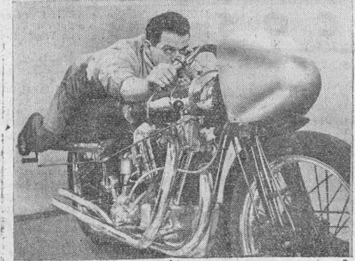
Bob Berry, que aparece en esta fotografía, en extraña postura sobre su máquina, es un famoso as de la velocidad británico, que va a intentar batir el récord de velocidad mundial en motocicleta. Para ofrecer menor resistencia al aire se protegerá tras esa espaciosa coraza aerodinámica y los pies, marcharán apoyados como muestra la fotografía. (Foto Calpe)
