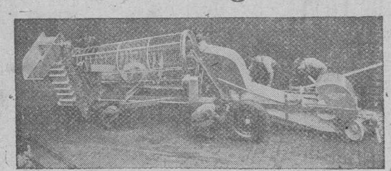
Máquina para la recolección de patatas construida por una fábrica británica. Para su manejo no se precisa más que un hombre y puede levantar 1.62 Has. de terreno al día. — (Foto CALPE.)
