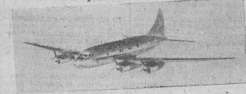
He aquí uno de los últimos tipos de avión para las necesidades del transporte civil: el "Avro Tudor I". Va equipado con cuatro motores Rolls Royce Merlin, su velocidad es de 300 millas por hora y su radio de acción de 4600.
