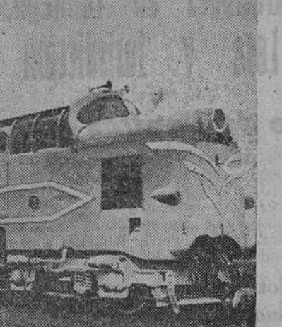
Londres.—Desde primeros de este mes de Noviembre, presta regularmente servicio de pasajeros entre Londres y Liverpool, un tren arrastrado por esta potente locomotora diésel eléctrica de 3.500 H. P. de potencia. Pesa 106 toneladas y su velocidad es de 90 millas por hora. La locomotora más potente de este tipo era la norteamericana con 2.400 H. P. (Foto Gil del Espinar)
