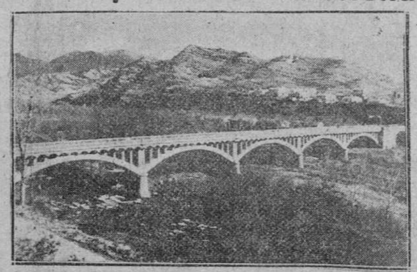
Una vista del nuevo puente sobre el Ter, en San Vicente de Torelló, provincia de Barcelona, inaugurado recientemente. Mide de largo 204,50 metros, con cinco arcos de 30 metros de luz y uno de 20; de alto, 13,50 metros y la anchura de la calzada es de 6,50 metros. — (Foto Gil del Espinar)
