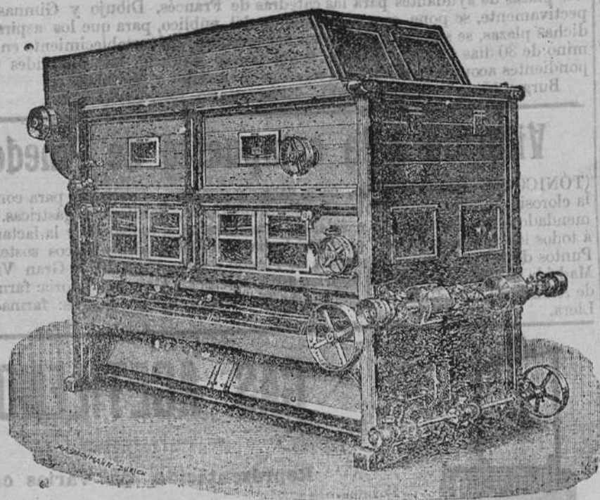
COLUMNA DESPUNTADORA
