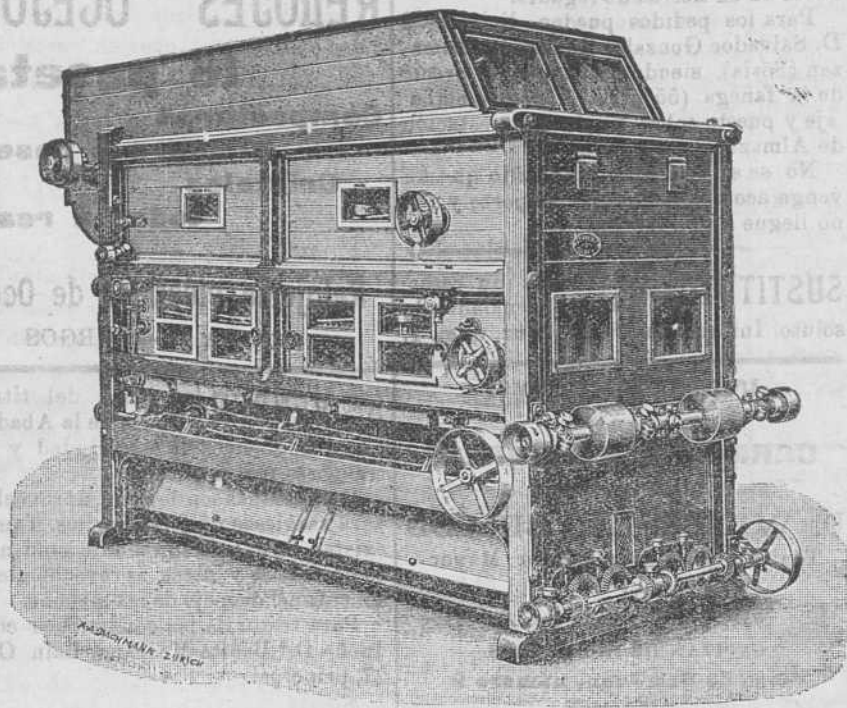
COLUMNA DESPUNTADORA
