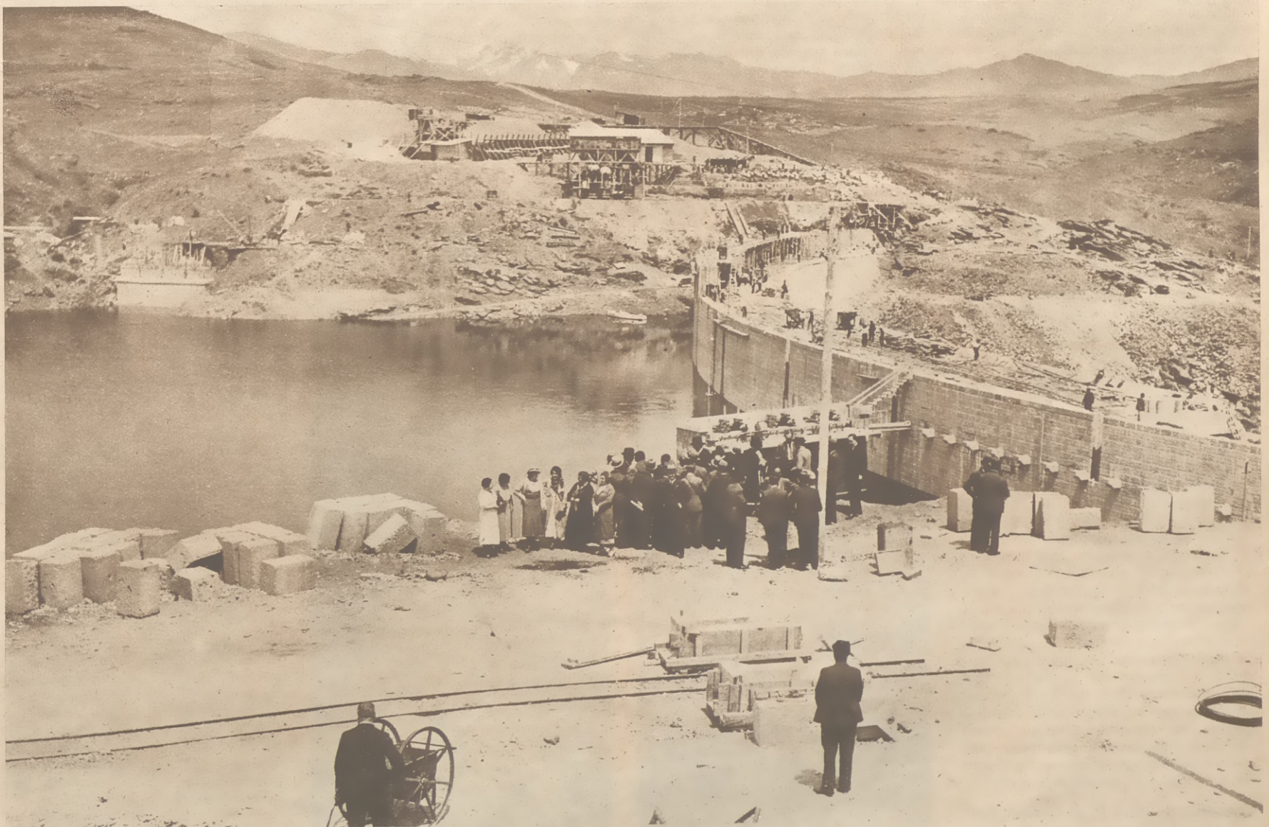
Las obras del embalse y la presa de Puentes Viejas, en el Canal del Lozoya
