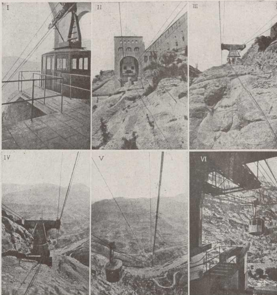
1. La cabina a l'estació superior. — 2. L'anden de l'estació superior. — 3. El castellet N.º 1. — 4. Una altra vista del mateix castellet. — 5. La cabina suspesa en el gran vano. — 6. La cabina entrant a l'estació inferior, prop del Llobregat.
