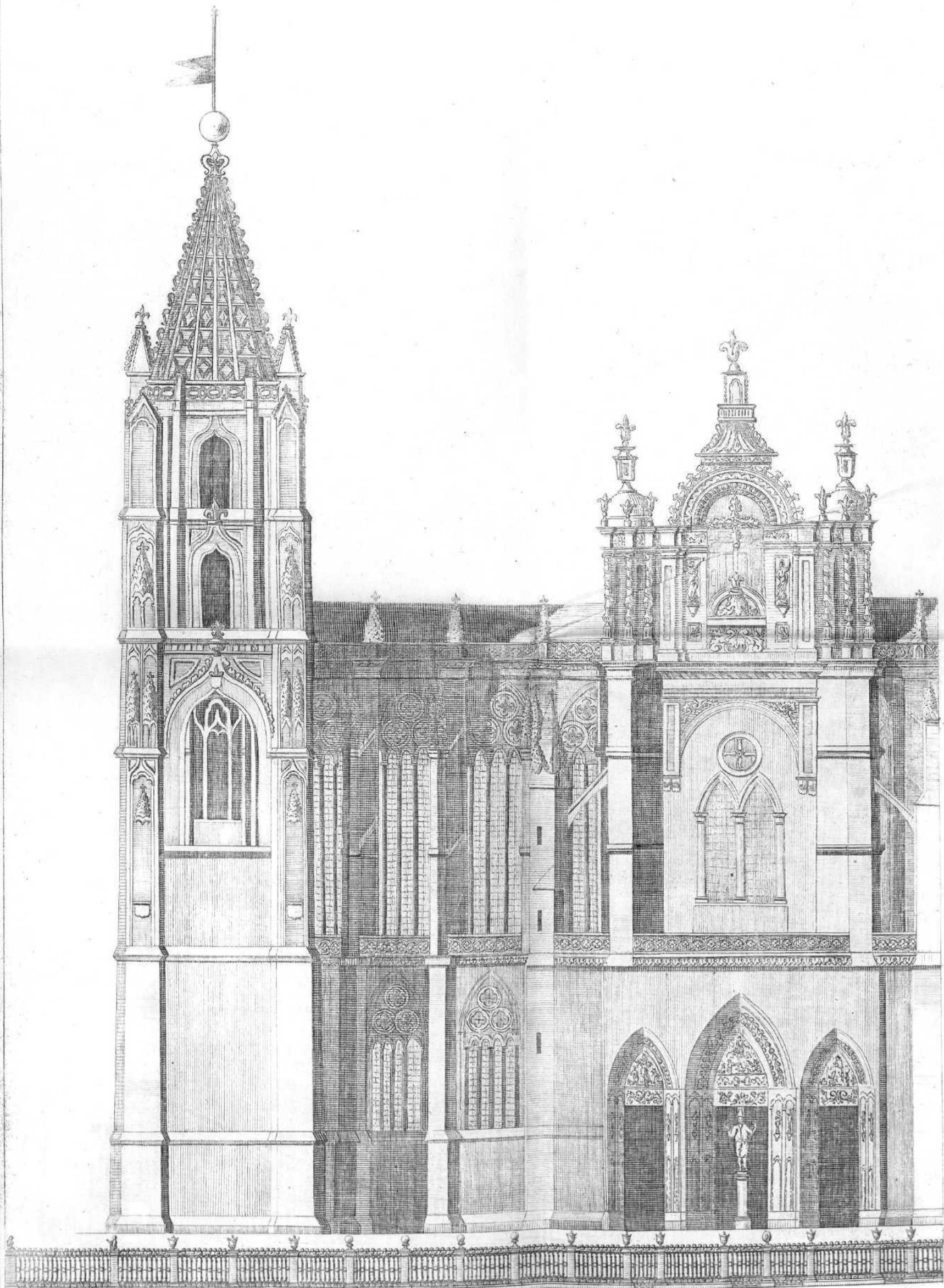
Ortografía de la fachada al mediodía de la S. ta Iglesia de Leon.
