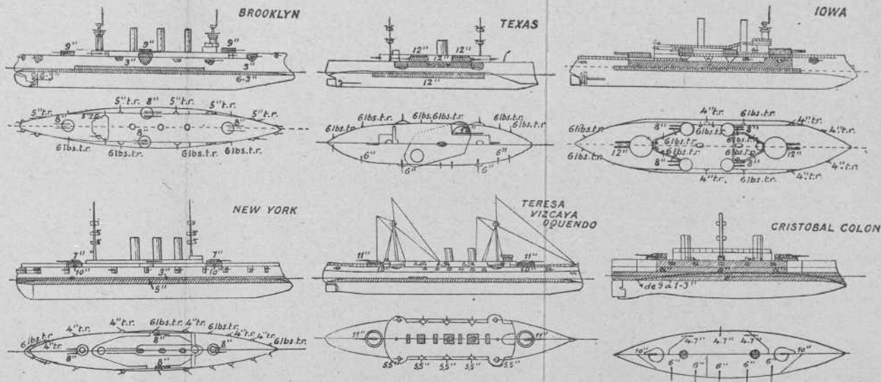
Plano y elevación del Brooklyn, Texas, Iowa, New-York, Maria Teresa, Vizcaya, Oquendo y Cristobal Colon.
