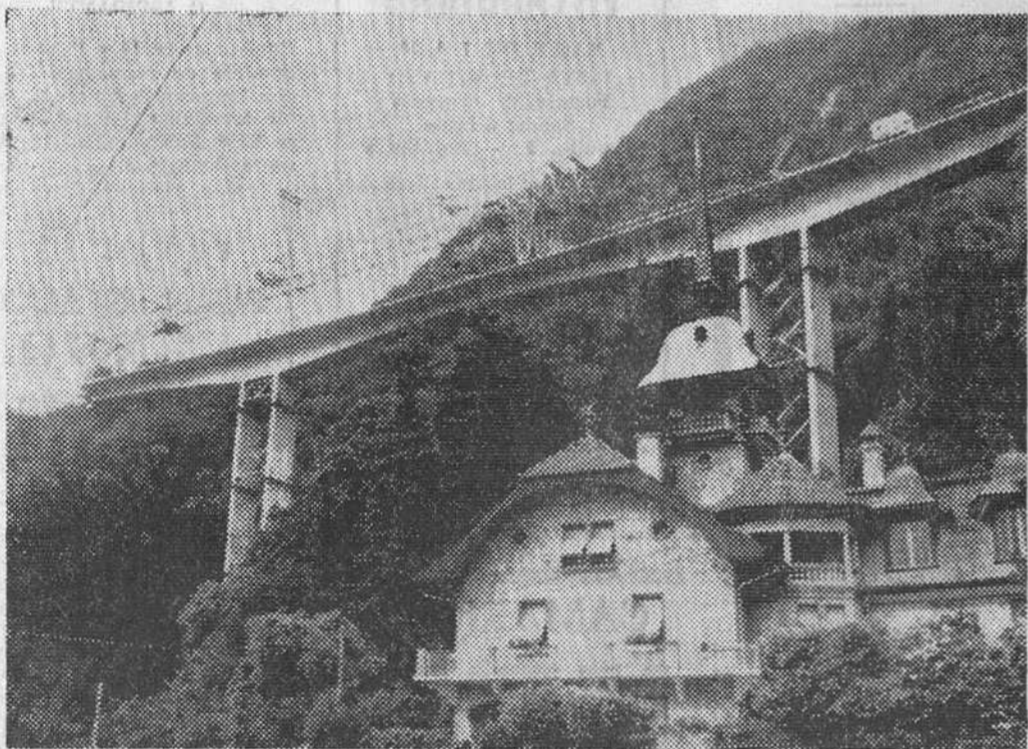
Un impresionante viaducto que permitirá a los automovilistas «sobrevolar» Montreux y el Castillo de Chillon, está siendo construido a toda prisa junto al lago Lemán. En esta foto vemos un aspecto de esta autopista. — (Foto FIEL)
