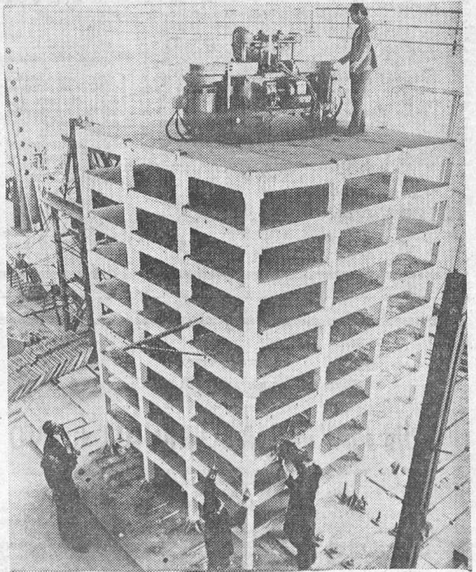
Todos los edificios de muchos pisos que se construyen en las repúblicas del Asia central, zonas de actividad sísmica, reciben sacudidas de hasta nueve grados. Por ello, en la base experimental del Instituto Científico Zonal de proyección de edificios residenciales y públicos, en Tashkent, capital de Uzbekistan, los modelos de las futuras edificaciones se someten al efecto de "Terremotos" artificiales, como el que vemos en la fotografía. — (Foto FIEL).
