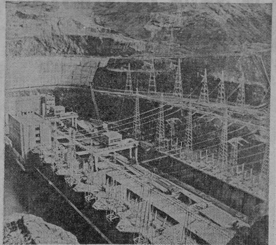
Moscú. — Las instalaciones hidroeléctricas de Nurek, en la región de Tajik, han empezado a funcionar, anticipándose a la fecha prevista. Es la octava unidad generadora de energía en funcionamiento, con capacidad para 2.400.000 kilovatios y se prepara ya la novena unidad, que comenzará también a producir, en breve. Estas instalaciones son las mayores del Asia Central. — (Foto FIEL-TASS).
