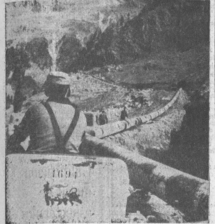
Al puerto de Génova ha llegado el primer barco cisterna con petróleo bruto que, a través del oleoducto Europa central, terminará en las refinadoras del Po (Italia), Aigle (Suiza) e Ingolstadt (Alemania), esta última a punto de terminarse. En la foto, una vista del oleoducto, en su fase final, atravesando los Alpes a 2.000 metros de altura. — Foto Fiel.
