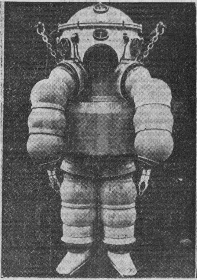
Aunque parezca un mariano no lo es. Dentro del traje metálico y cerrado herméticamente va un hombre: el buzo. Un hombre que hace su vida en las pintorescas pero también peligrosas profundidades marinas. Con este extraño traje se pueden soportar presiones de hasta sesenta atmósferas y descender a 170 metros de profundidad.
