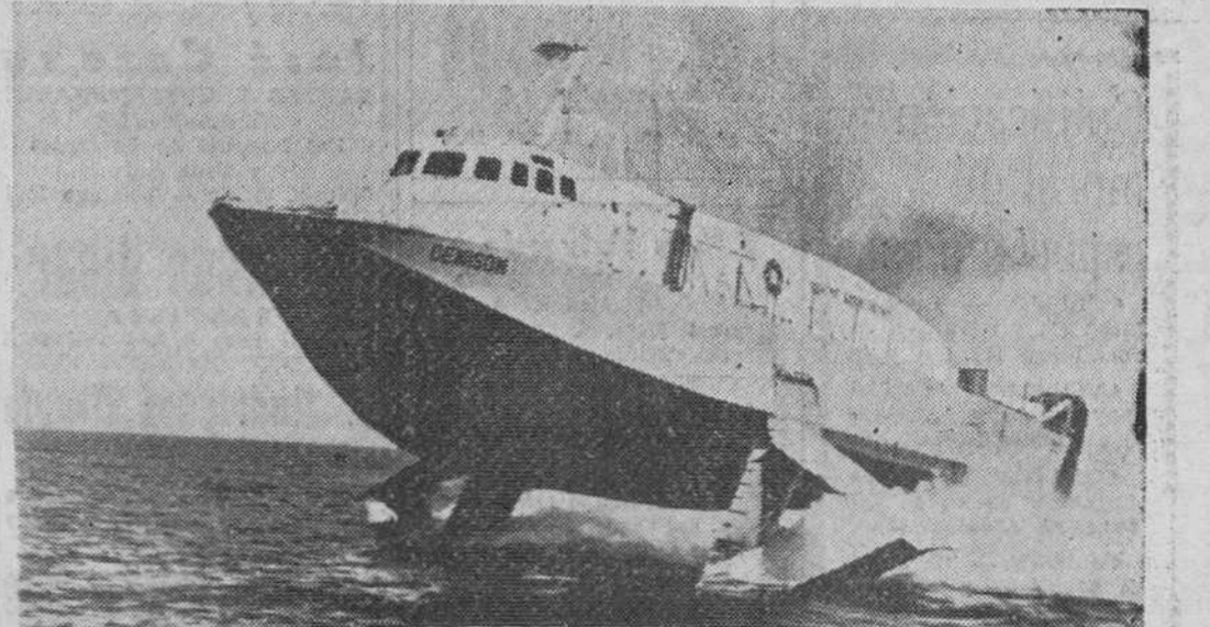
Durante un viaje de pruebas, vemos al primer prototipo de chidrofili oceánico, el «Denison», que ha alcanzado velocidades de 55 nudos sobre olas de 2,70 metros de altura. Las pruebas tuvieron lugar en aguas de la Academia de la Marina Mercante de los EE. UU. y el prototipo servirá para estudiar las posibilidades operacionales de los chidrofili de mayor tamaño, en aguas del océano.—(Foto FIEL)
