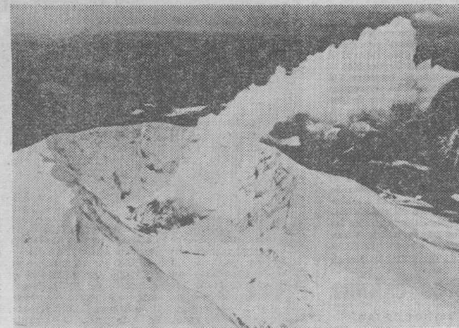
Monte Santa Helena (Washington). — Numerosos vapores son expulsados del cráter del Monte Santa Helena, que ha sido visitado recientemente por unos científicos y en el que han notado una subida en el nivel del suelo, lo que podría suponer que, en cualquier momento surgiera del volcán una leve erupción. — (Telefoto Efe-AP)
