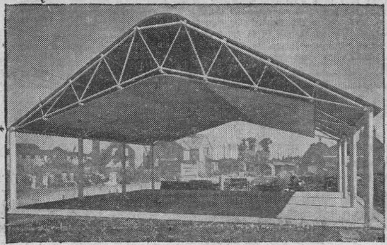
En Gran Bretaña se han construido estos originales tejados destinados a los países tropicales. Son de fácil transporte y montaje y su coste es reducido.—(Foto Calpe)
