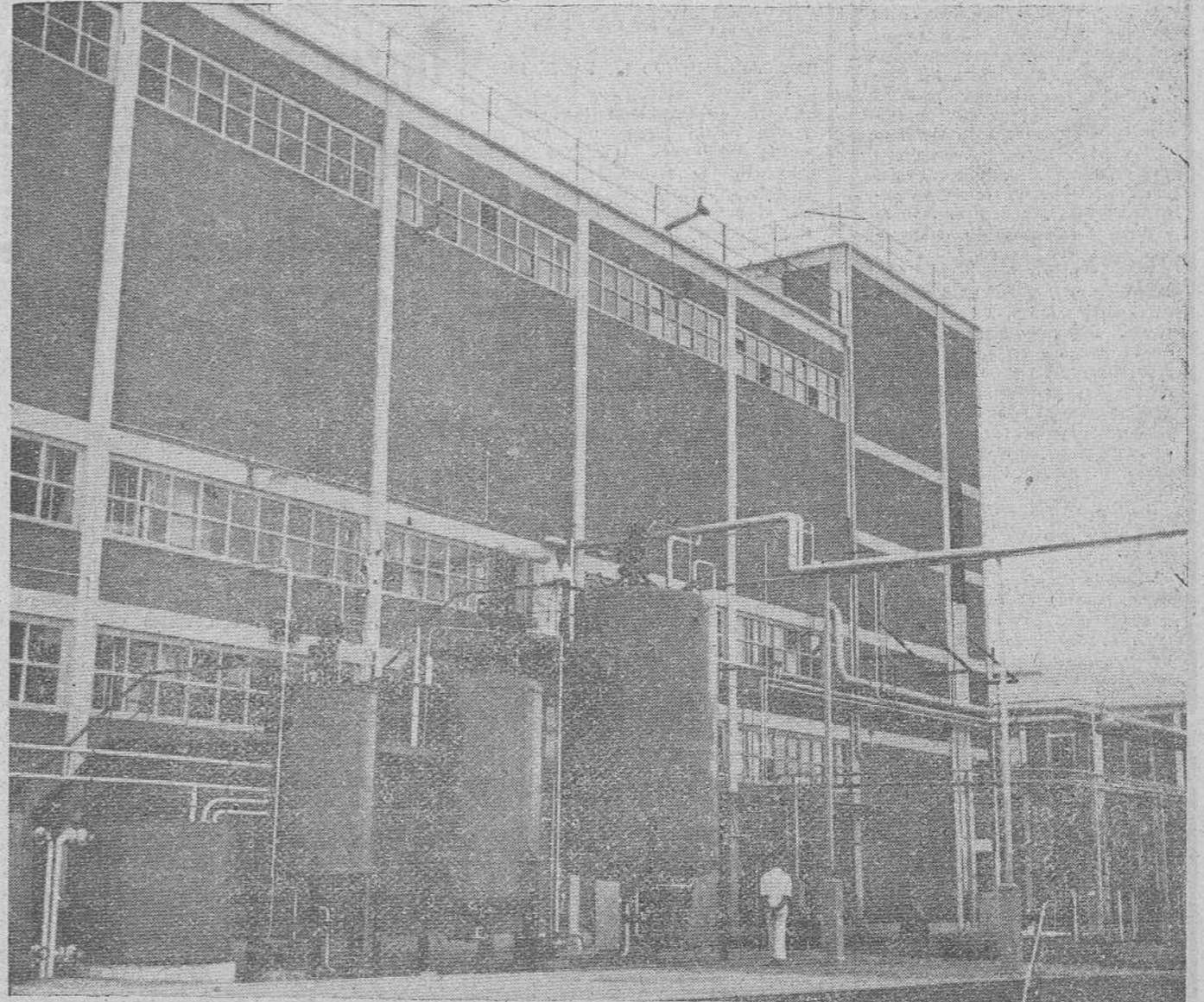
Conducciones exteriores de la fábrica de estreptomicin
