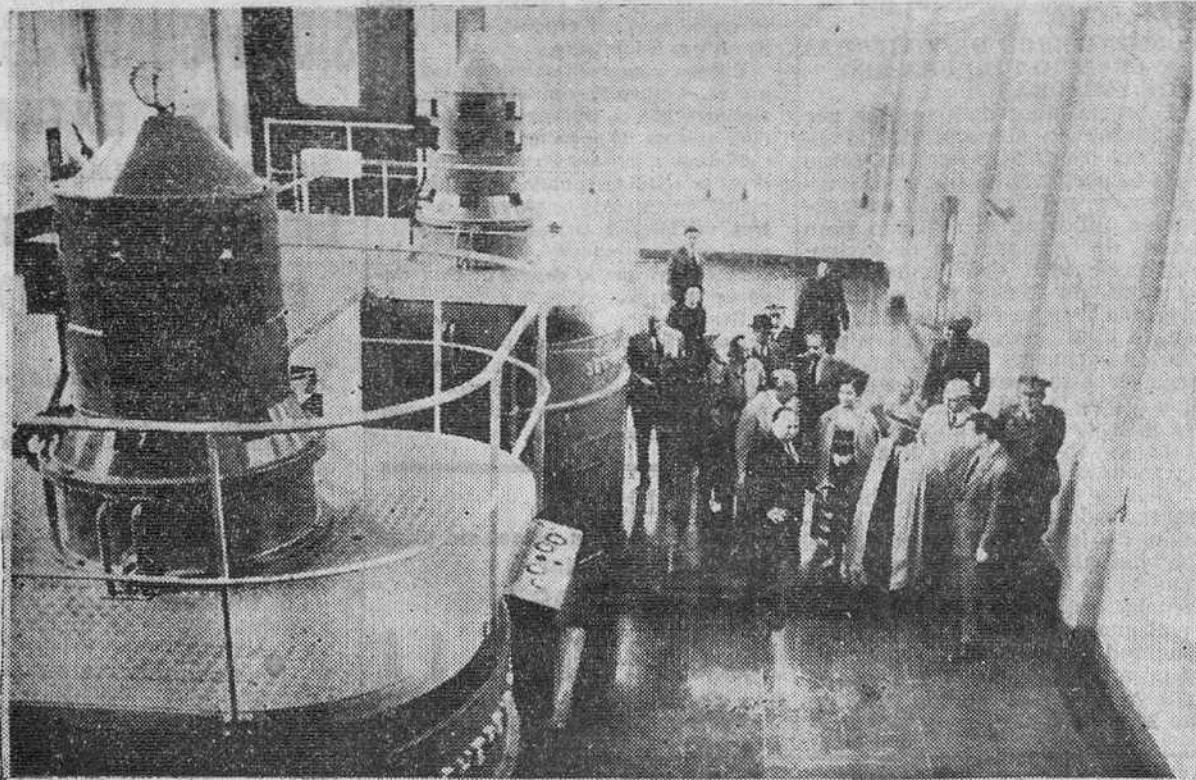
S. E. el Jefe del Estado inaugura la central eléctrica de Bono, cuya potencia en turbina es de 5.500 CV. y la capacidad de alternadores de 3.800 KW. en su visita a la cuenca del Ribagorzana. — (Foto Cifra)
