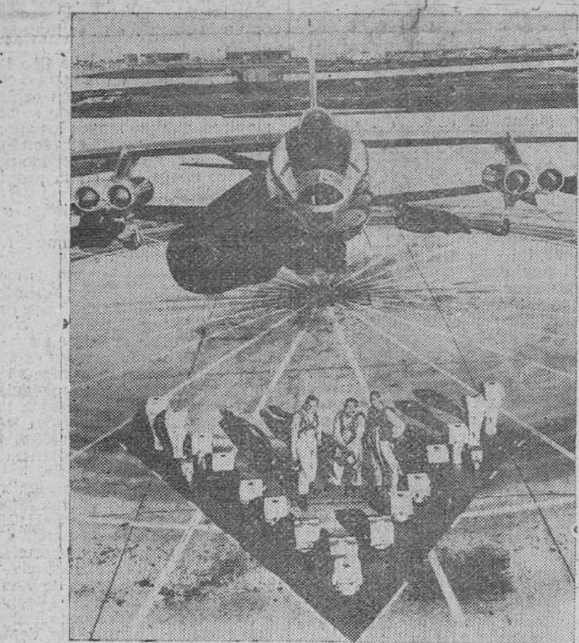
Las fotografías que aparecen de arriba a abajo y de izquierda a derecha, reproducen: un avión norteamericano RB-47 de reconocimiento medio, que tiene una tripulación de tres hombres, y lleva siete cámaras que pueden funcionar simultáneamente en vuelo. Este avión puede fotografiar millón y medio de kilómetros cuadrados en tres horas.
