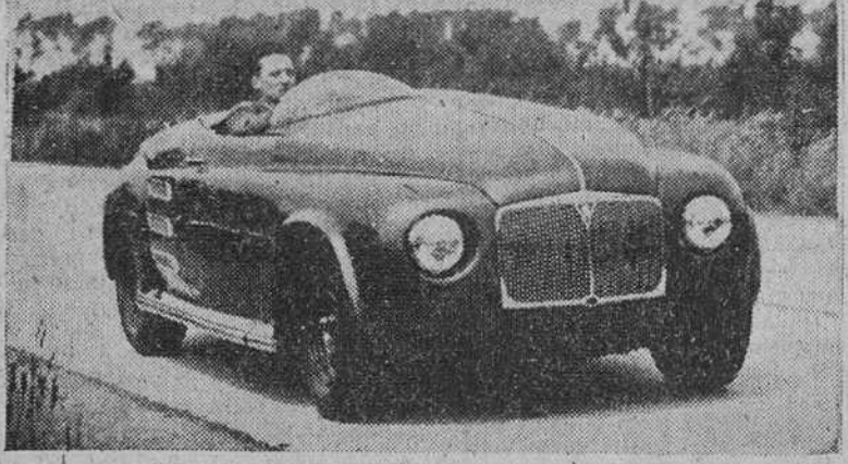
El "Rover" de turbina de gas. Se aprecia la entrada de aire en la parte posterior del vehiculo.
