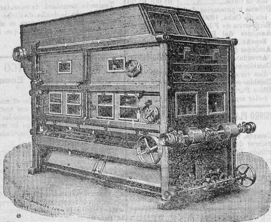
COLUMNA DESPUNTADORA
