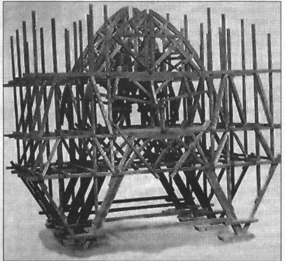
Esquema de encimbrado de una bóveda
