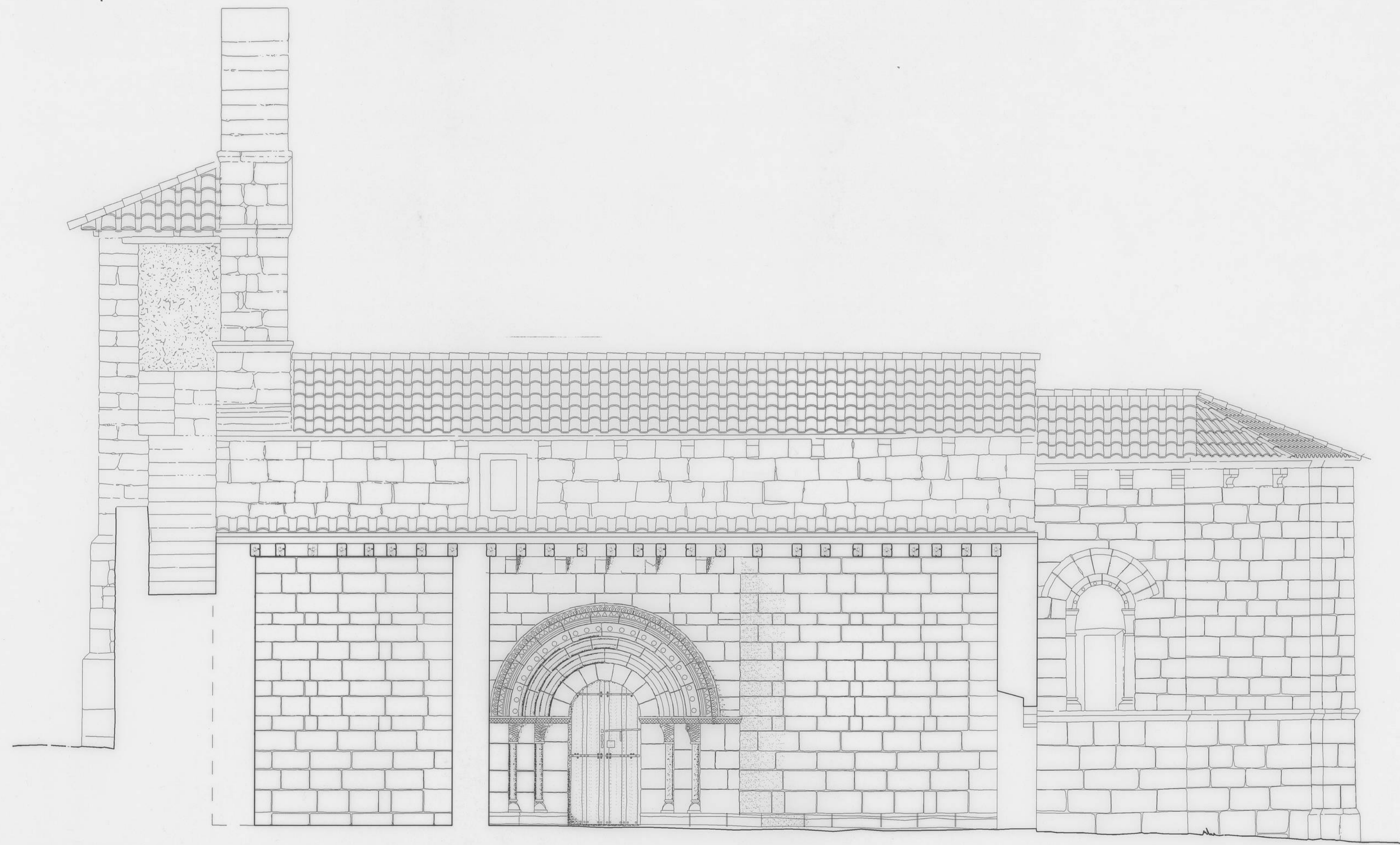
SECCION LONGITUDINAL LADO SUR
