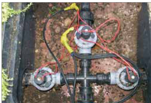
3.11: electroválvulas. Nos permiten regar y/o fertilizar los sectores del huerto que deseemos
