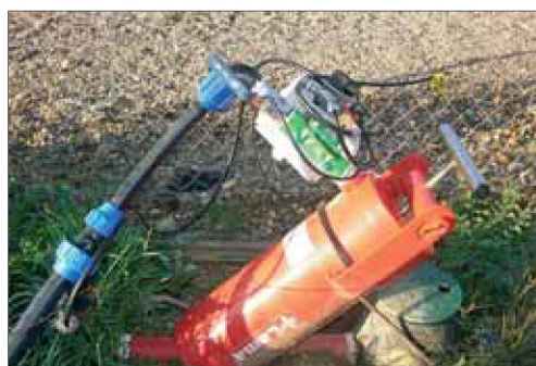
3.10: se hace pasar al agua de riego por el tanque que tiene el fertilizante disuelto. Antes de distribuirse, pasa por un filtro por si pudiera tener algún elemento que nos obstruya las boquillas del riego
