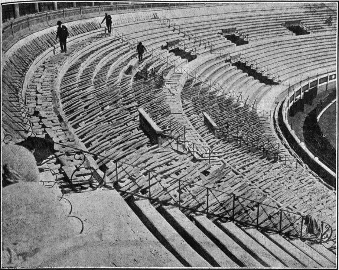
ASPECTO DEL TENDIDO EN QUE SE INICIÓ EL HUNDIMIENTO, DURANTE LA PRUEBA DE RESISTENCIA
