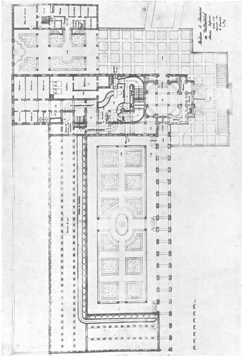
Lám. V.—Archivo de Simancas en Valladolid. Planta inferior.
