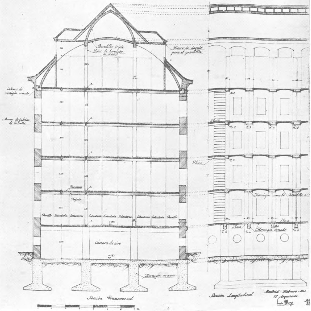
Lám. VII.—Archivo de Simancas en Valladolid. Detalle del depósito.
