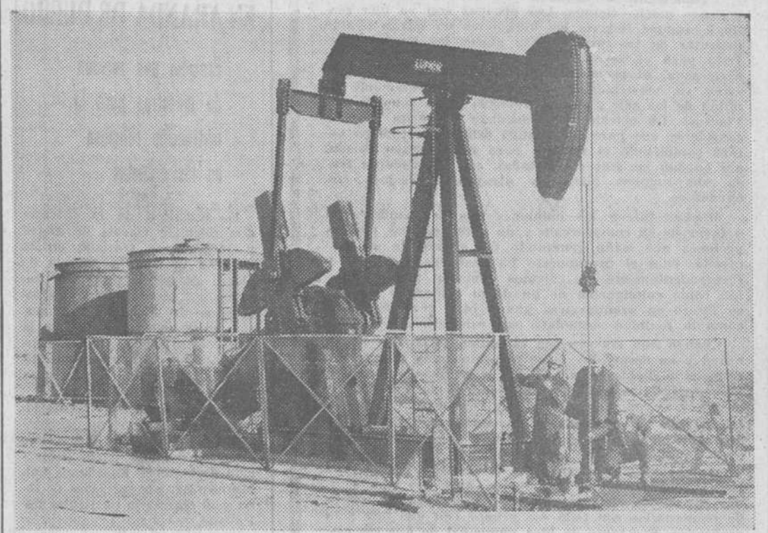
El «Hontomin 2» comenzó ayer a producir petróleo del Jurásico a base de bomba de balanceo. Esta producción que se hace a título experimental, sigue a las pruebas de pistoneo que dieron un rendimiento diario de 200 barriles de crudo. En nuestro grabado puede verse la estructura metálica de la cabeza de caballo articulado tal y como fue captada por la cámara de nuestro fotógrafo. La duración de esta nueva fase de trabajos de producción depende de los medios de evacuación del crudo y de la solución técnica que vaya a darse a su destino comercial. (Foto FEDE)
