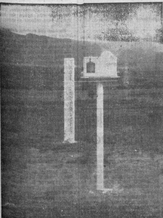
Actinógrafo instalado en la estación meteorológica.
