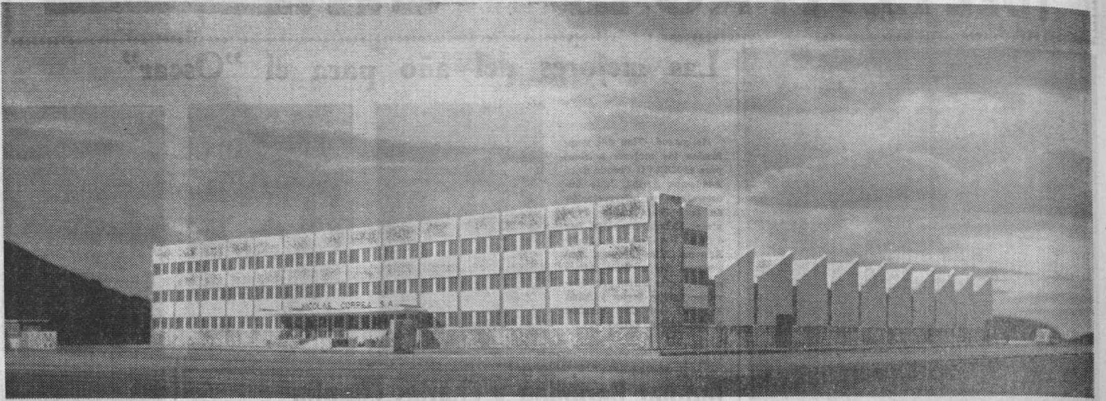
Aspecto actual de las obras de «Nicolás Correa, S. A.», sin duda la primera fábrica de nueva planta que será inaugurada dentro del «Polo»
