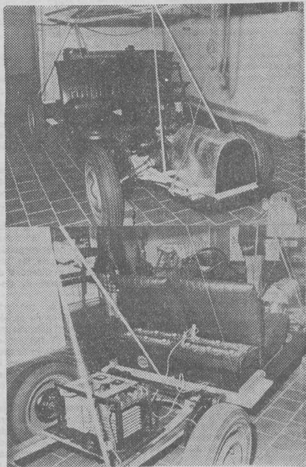
Un modelo de automóvil solar. Las baterías situadas detrás de los asientos sirven para almacenar la energía suministrada por la gran pantalla que capta los rayos de sol. — (Foto EFE-FIEL)
