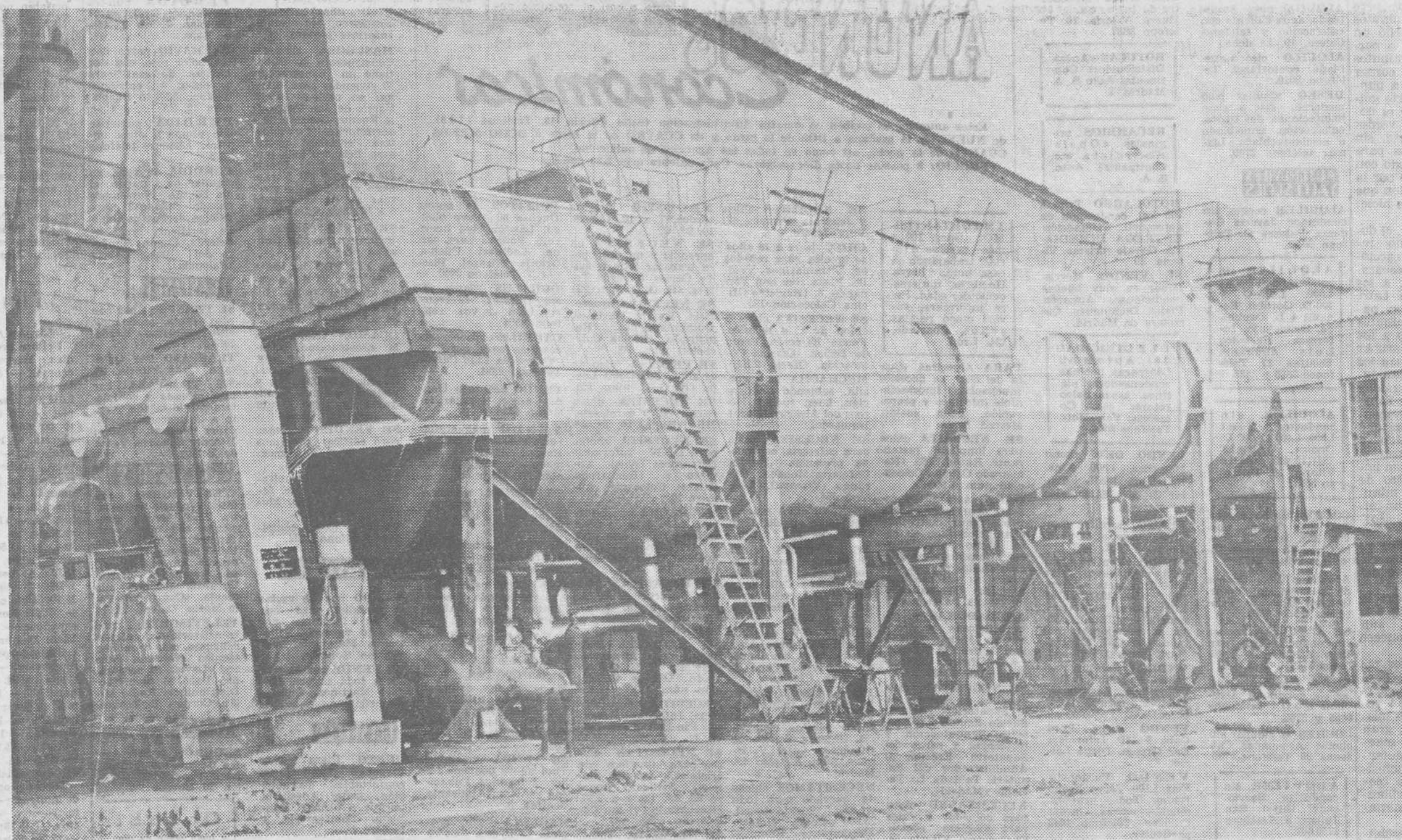
Primera difusión DDS instalada en España. Ha sido montada en el exterior de la factoria de EBRO Cia. de Azúcares y Alcoholes en Toro.
