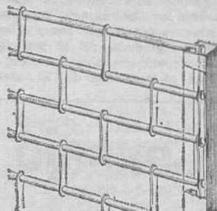
Modelo «ÁLUACERO» Detalle de seguridad
