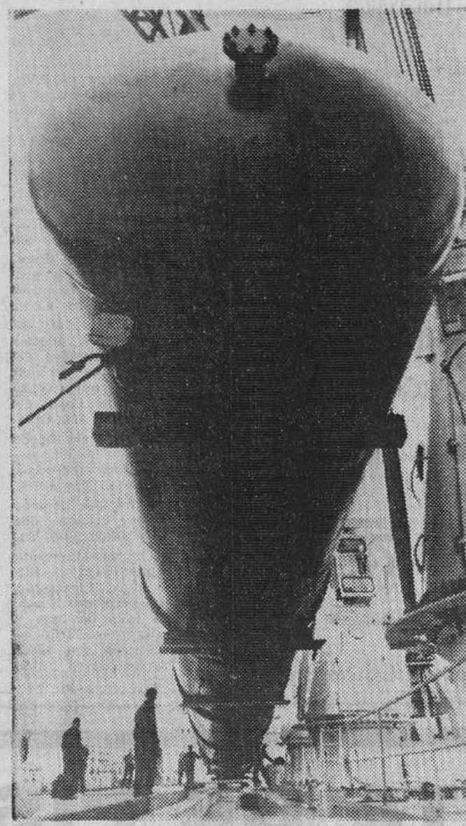
Más de 33 metros de largo y tres de diámetro mide este gigantesco «cigarro» de 60 toneladas que una enorme grúa instala sobre la cubierta del carguero «Trinidad» en el puerto de Hamburgo. Se trata en realidad de una enorme pieza para la industria química en Filipinas. Tres semanas de viaje tardará en llegar a su destino. — (Foto FIEL)
