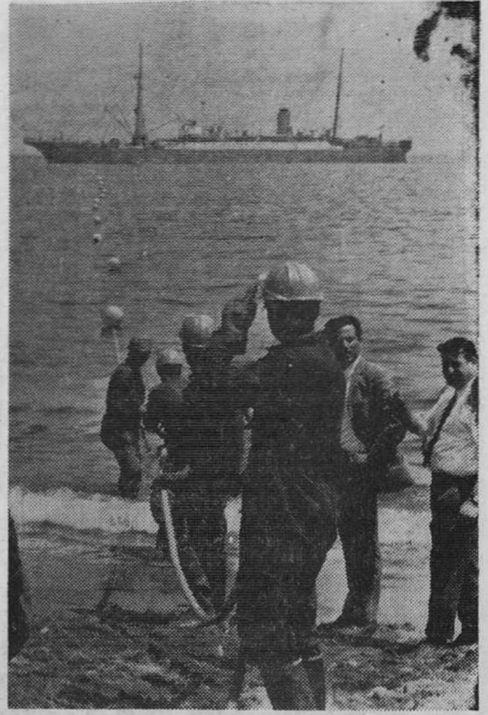
Frente al Paseo Marítimo de Barcelona han dado comienzo los trabajos de tendido de un cable coaxial submarino para la unión telefónica de Barcelona y Pisa (Italia).
