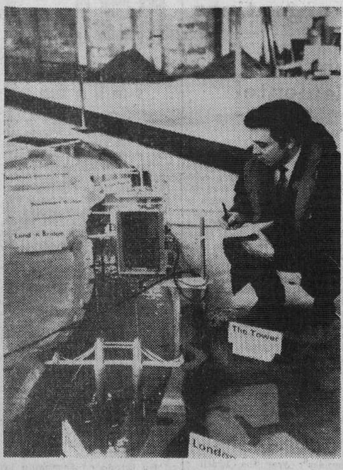
Un técnico en hidráulica inspecciona la altura del agua, por medio de un aparato medidor de niveles, en una de las secciones de 385 pies de longitud que en forma de maqueta existe en la Estación de Investigación Hidráulica del Ministerio británico de Tecnología, para la prevención y protección de Londres de peligrosas inundaciones. Cada siglo el mar del Norte aumenta en trece pulgadas y Londres disminuye en doce. Esto, unido a la cada vez mayor cantidad de ciénega en el fondo del Támesis, hace que el peligro de las inundaciones sea un problema a estudiar con gran interés (Foto FIEL)
