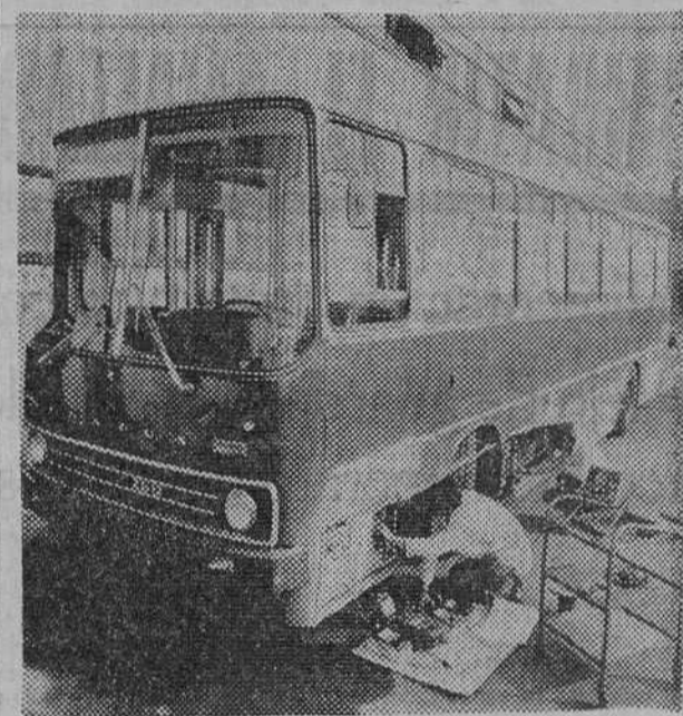
En la Institución de Investigación Eléctrica, de Budapest ha sido construido un motor de coche que funcionará con Diesel y con electricidad. El motor será instalado en el autobús modelo «LK-260 Irkus» y, si los resultados son satisfactorios, se utilizará en los transportes públicos de la capital húngara. (Foto FIEL)
