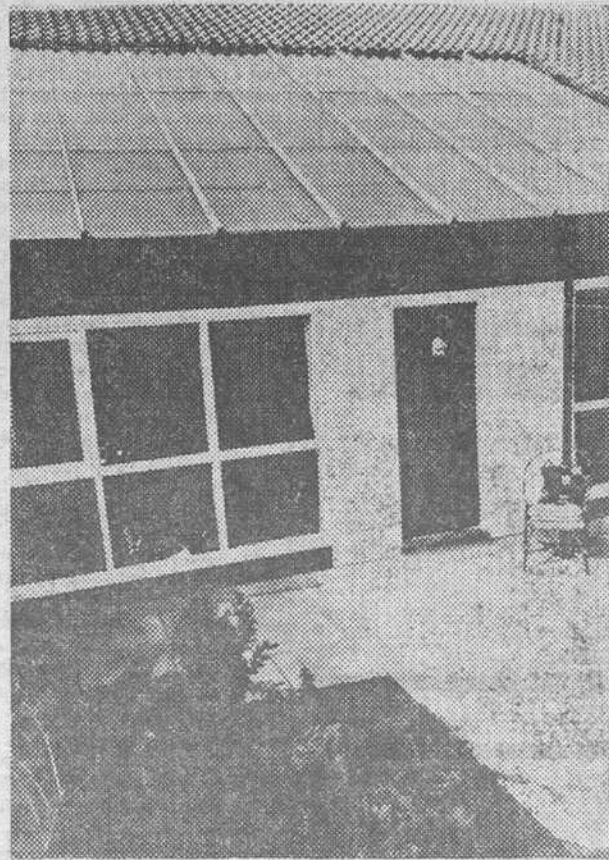
La casa solar de Milton Keynes. Una parte de las tejas ha sido reemplazada por placas de vidrio que protegen el colector de energía solar (Foto EFE-FIEL)
