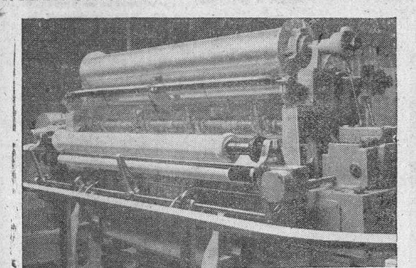
LOS INGENIEROS TEXTILES BRITANICOS HAN TERMINADO SUS EXPERIMENTOS CON ESTA NUEVA MAQUINA PARA GENEROS DE PUNTO QUE TRABAJA A UN RITMO DOBLE QUE EL DE CUALQUIER OTRA MAQUINA. CON ALGUNAS ADAPTACIONES LA NUEVA MAQUINA TAMBIEN PUEDE PRODUCIR MATERIAL DE PUNTO PARA VESTIDOS, BUFANDAS, B LUSAS Y PULLOVERS DE PUNTO.—(Galpe)
